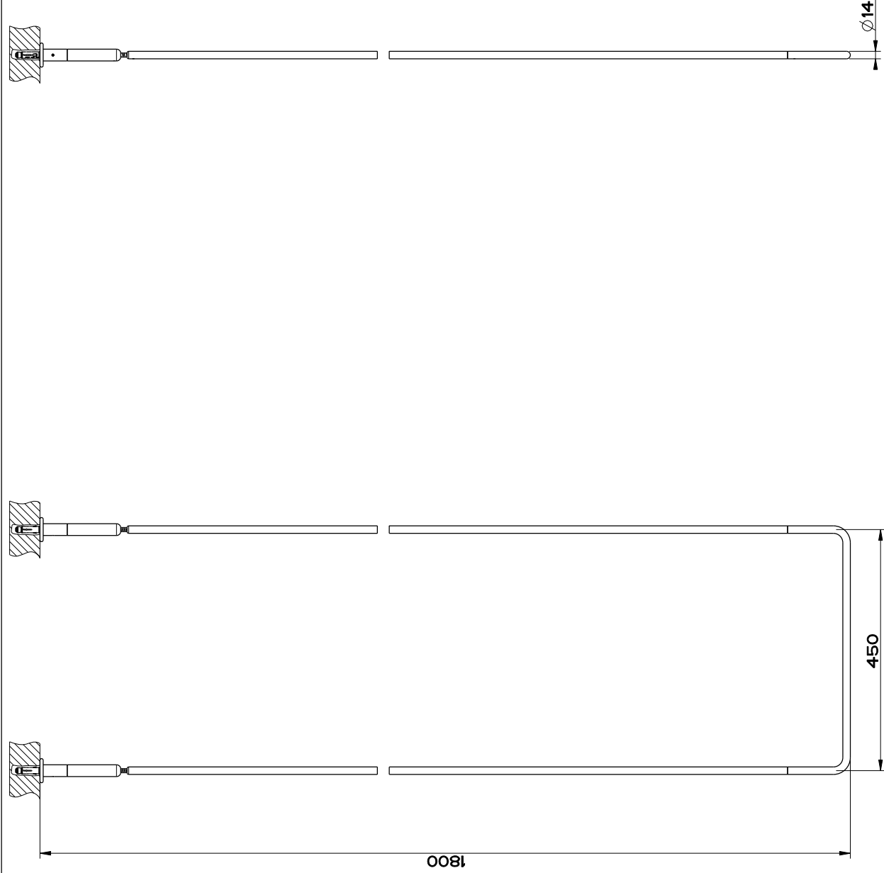
Montaggio su cartongesso con tasselli KD8 (ordinare a parte art.29724)
